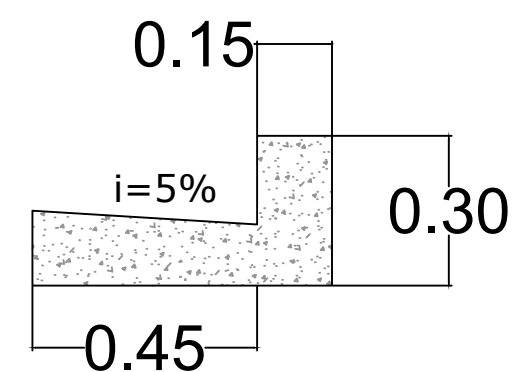
PAVIMENTAÇÃO ASFÁLTICA DET. GUIA E SARJETA
