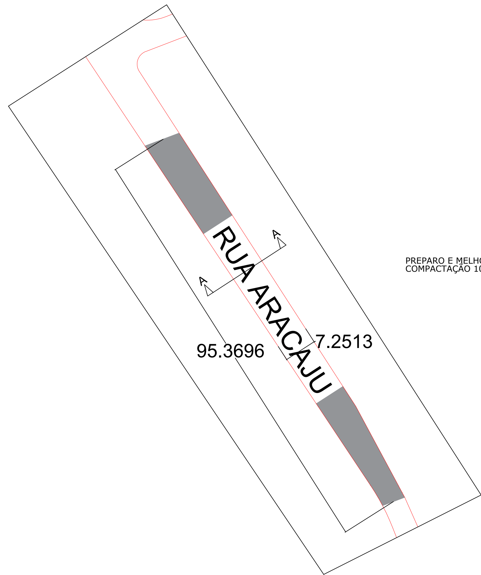
PAVIMENTAÇÃO ASFÁLTICA PLANTA BAIXA
