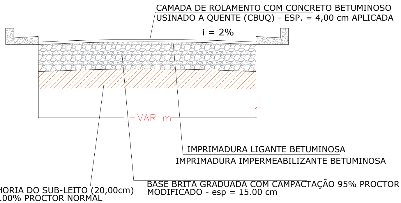
PAVIMENTAÇÃO ASFÁLTICA SEÇÃO TRANSVERSAL CORTE AA
